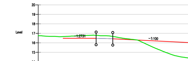
Alignment - SQS Entry SCALE: H 1:1000, V 1:200. DATUM: 14.000
